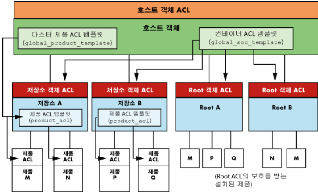
그림 9-2 ACL 템플릿
