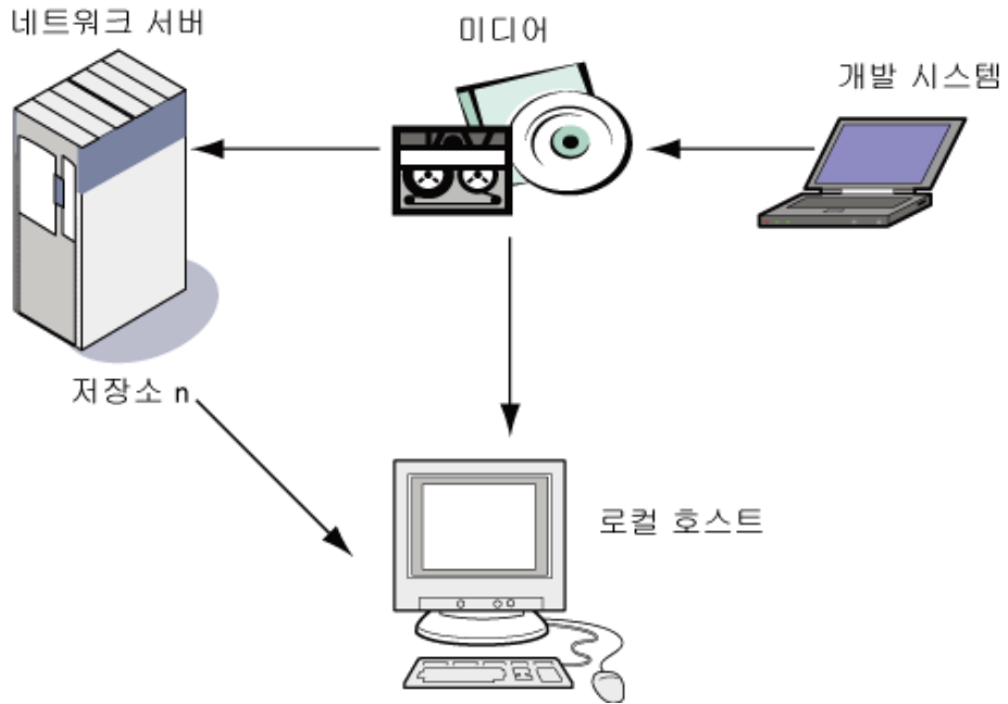
그림 1-1 SD-UX 시스템
