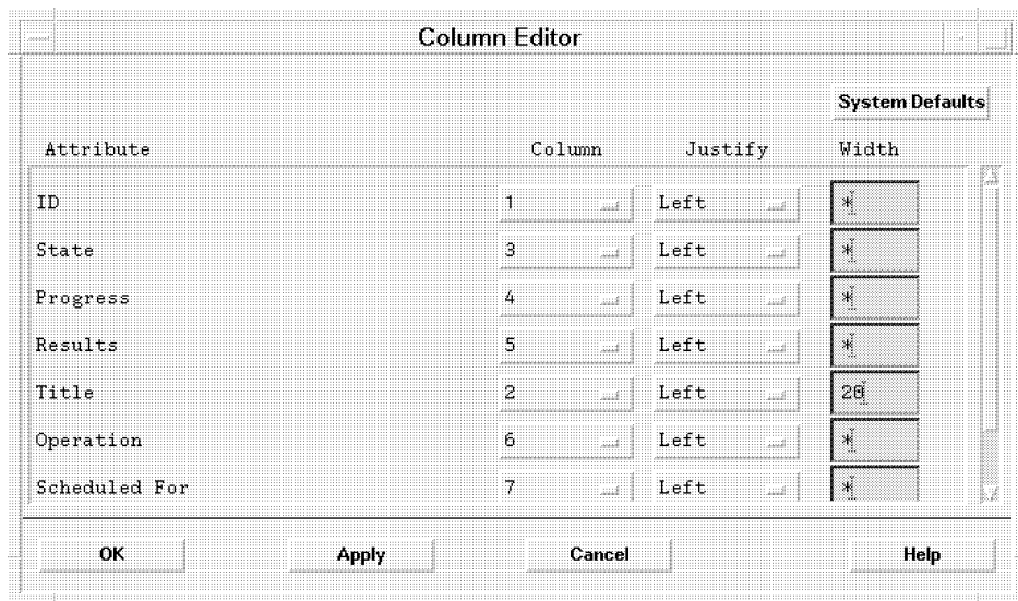
그림 1-6 Column Editor
